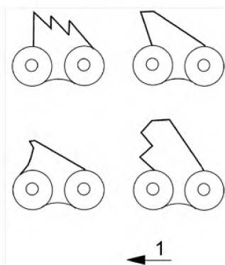
Рисунок С.3 – Вид спереди приемлемого профиля зуба цепи
