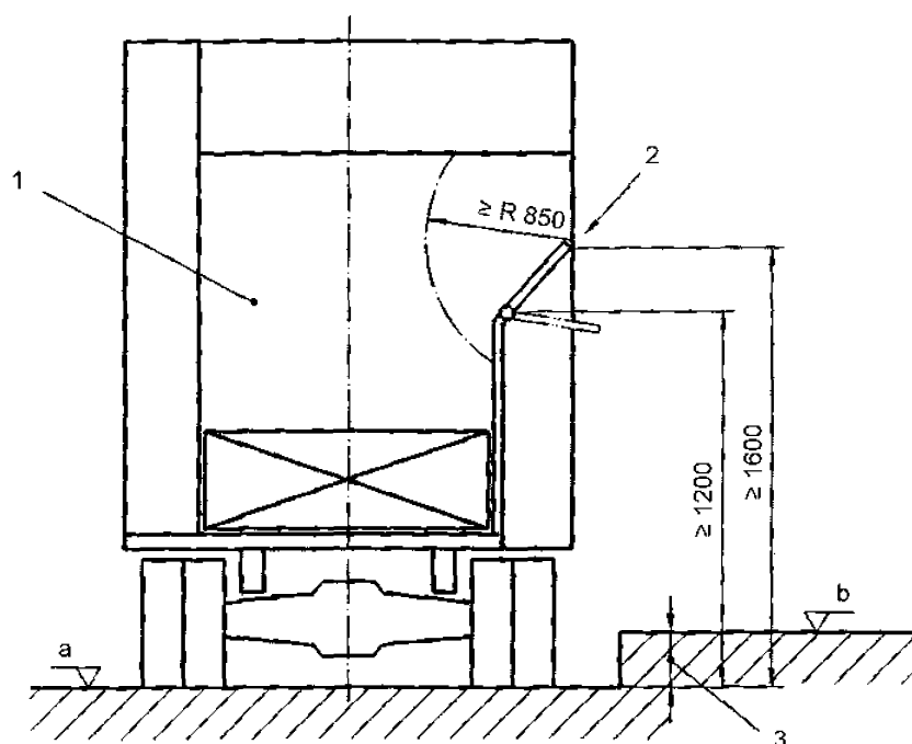
1 – бункер; 2 – силовая балка; 3 – стандартная высота бордюра, равная 200 мм; янки мусоровоза; b – бордюр
