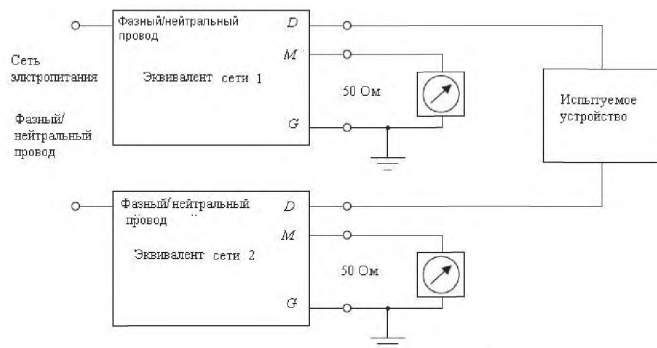
Топология схемы по EN 55016-1-2:2004, рисунок 4. Значения применимы к полосе частот от 3 до 9 кГц Рисунок 3 – Эквивалент сети от 3 до 9 кГц
