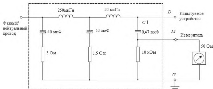
Топология схемы по EN 55016-1-2:2004, рисунок 4. Значения применимы к полосе частот от 3 до 9 кГц Рисунок 3 – Эквивалент сети от 3 до 9 кГц
