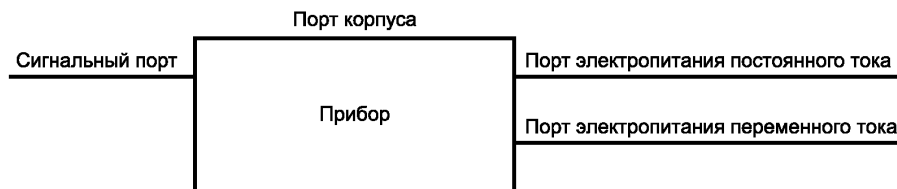
Рисунок 1 — Примеры портов
