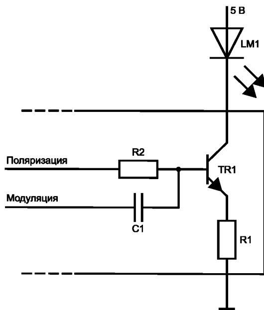
Рисунок D.2 — Задающий контур обычного лазера
