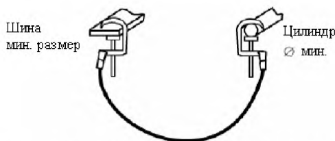
Рисунок 5с – Комбинация шины и цилиндра минимального размера
