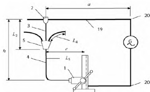
Рисунок 7d – Для испытуемого заземляющего кабеля в соответствии с рисунком 2а
