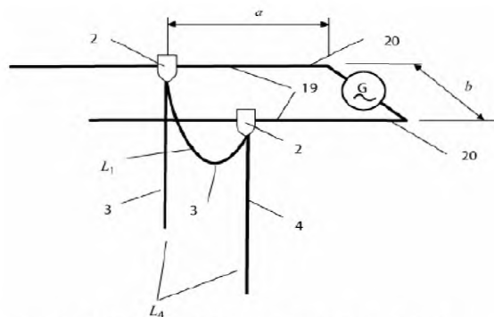
Рисунок 7с – Для испытательных устройств в соответствии с рисунками 2b и 2е
