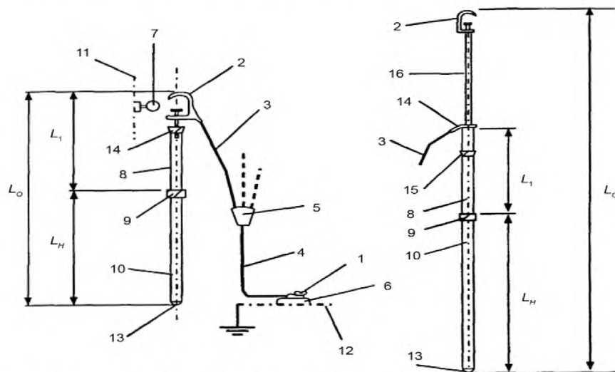
Рисунок 1а – Многополюсное оборудование
