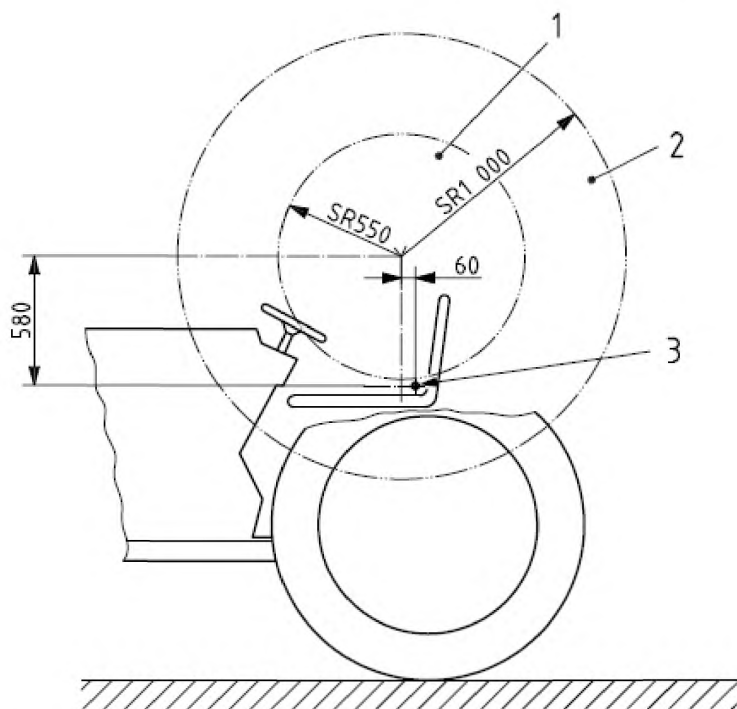
Рисунок 3 – Зона досягаемости рук оператора
