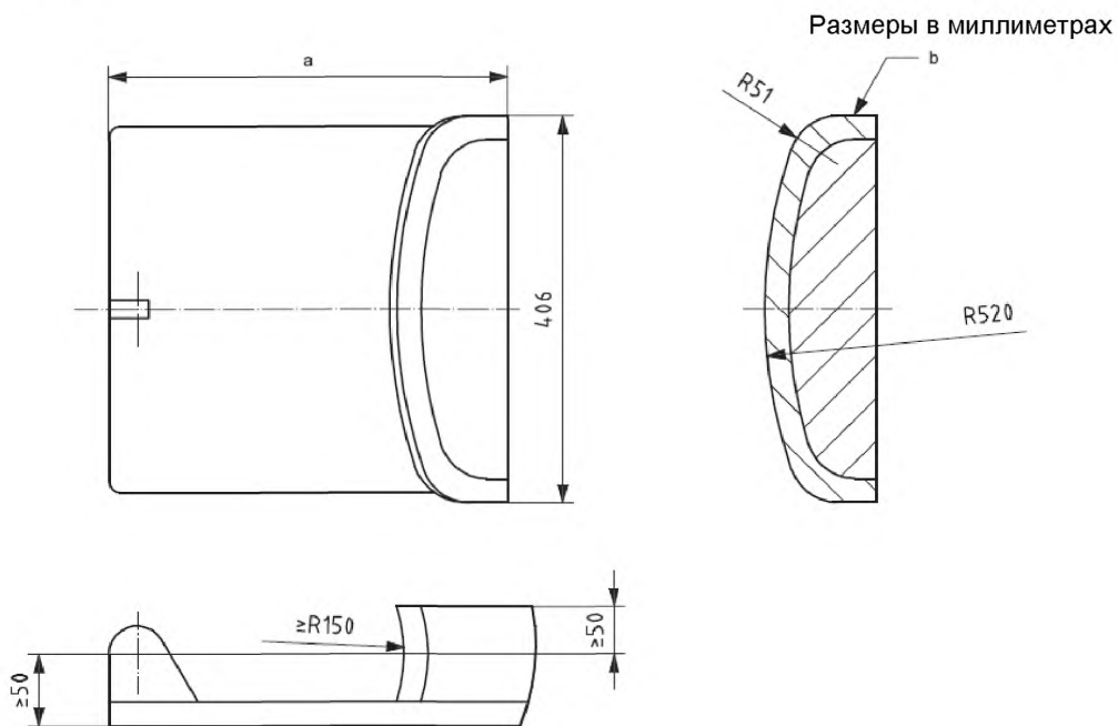
Рисунок 1 – Тяговое устройство
