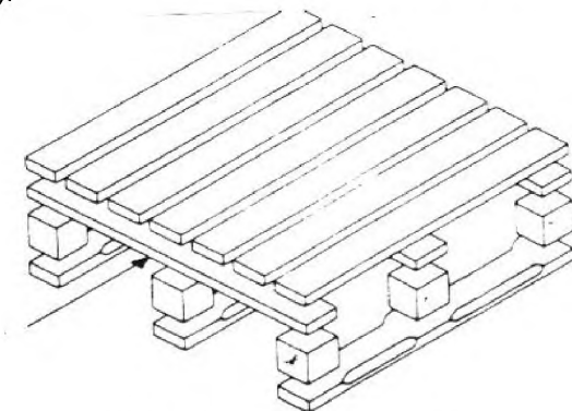
Рисунок 57 – Поперечная доска
