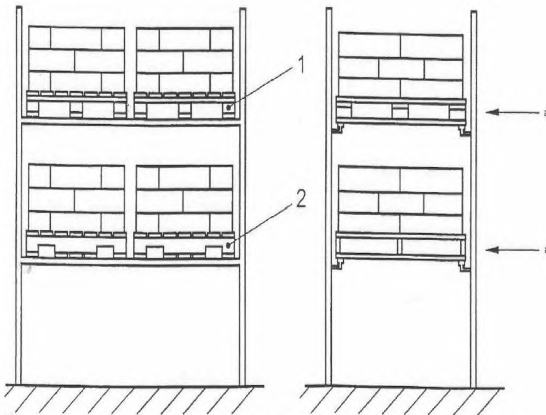
1 – четырехзаходный поддон со свободным заходом; 2 – поддон с продольной выемкой; а – сторона загрузки
