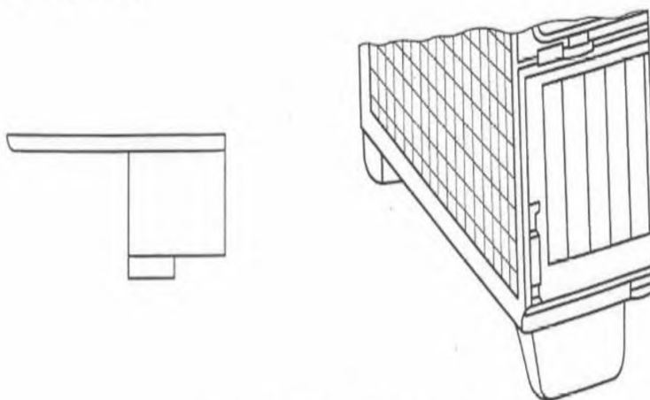
Рисунок 60 – Гнездовая опора
