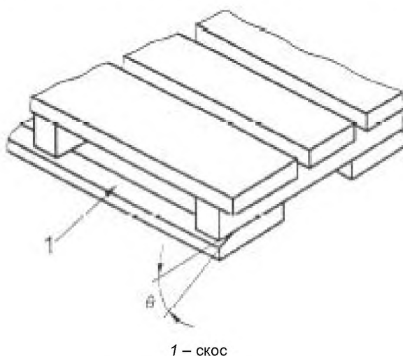
Рисунок 48 – Сплошной скос
