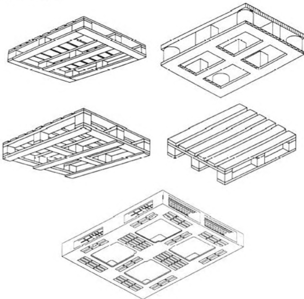
Рисунок 41 – Просветы поддонов
