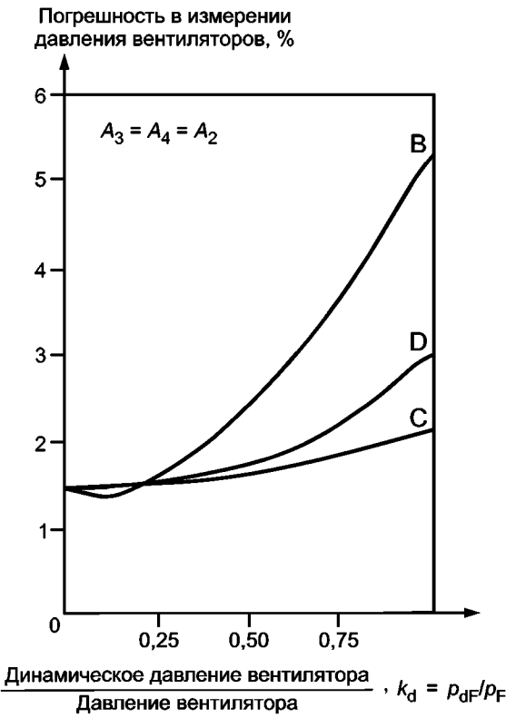
Рисунок 29 — Погрешность при измерении давления вентилятора
