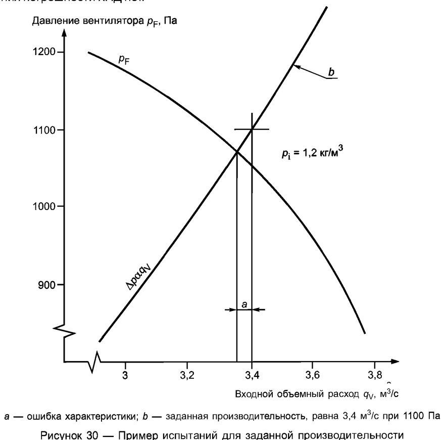
Рисунок 30 — Пример испытаний для заданной производительности
