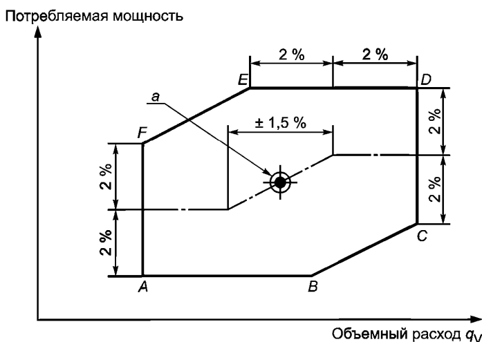
Рисунок 32 — Типичный пример зависимости погрешности мощности от объемного расхода
