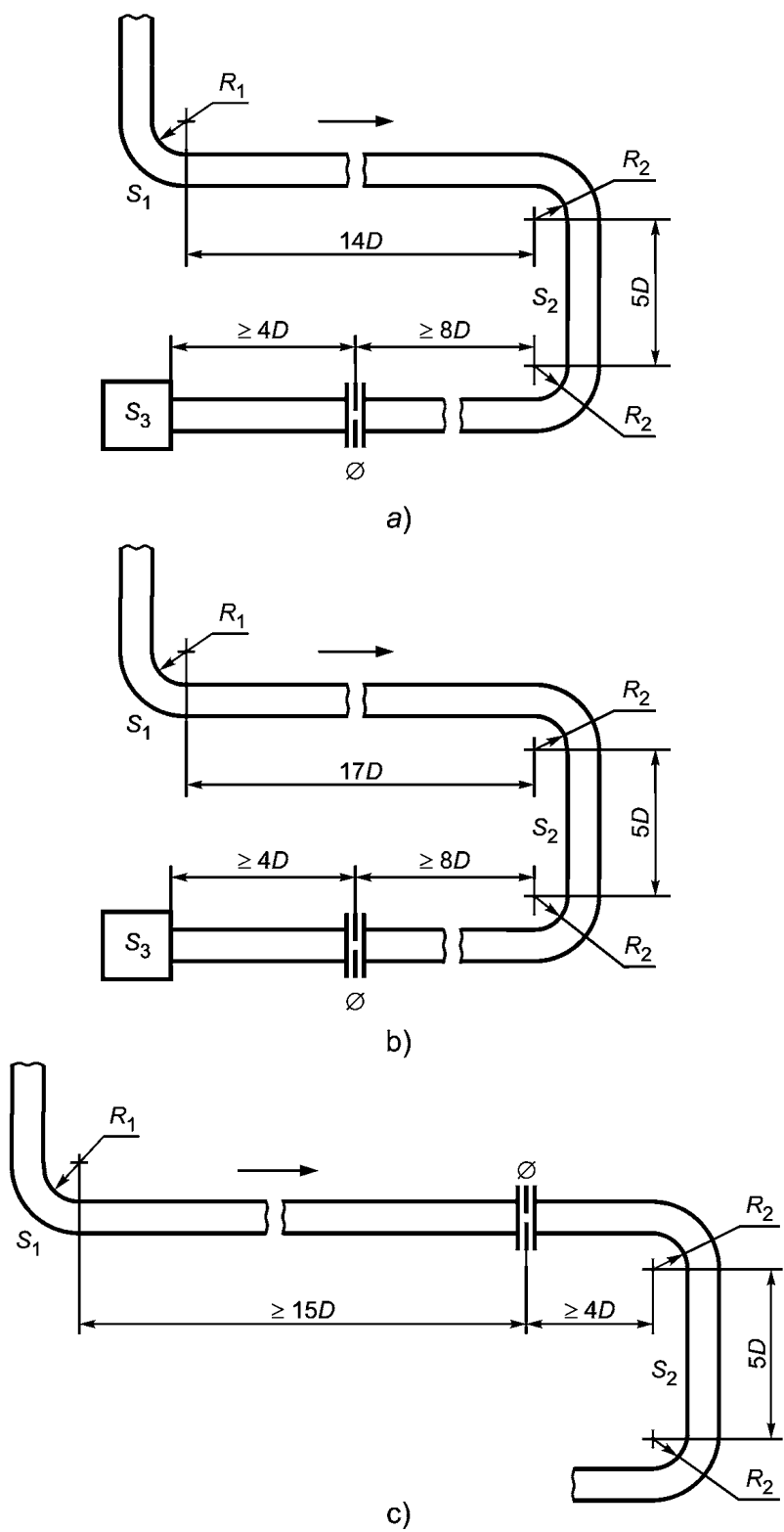
S_1 — поворот на 90^\circ , R/D = 1 ; \varnothing — измерительная диафрагма, r_A = 0,64 ; S_2 — двойной поворот на 90^\circ , R/D = 1,5 с промежутком 5 D ; \rightarrow — направление движения потока; S_3 — любой источник возмущения
