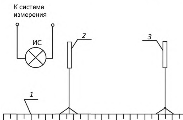
1 – фотометрическая скамья; 2 – штормы; 3 – фотоприемное устройство Рисунок И.1
