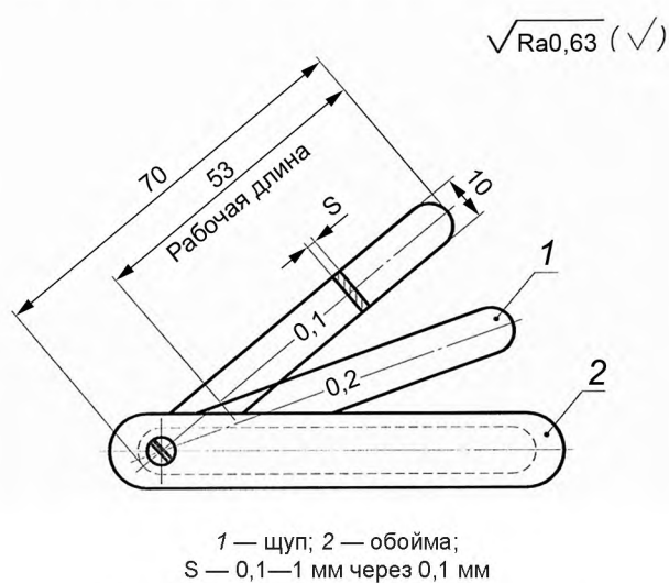
Рисунок Е.12 — Набор щупов плоских
