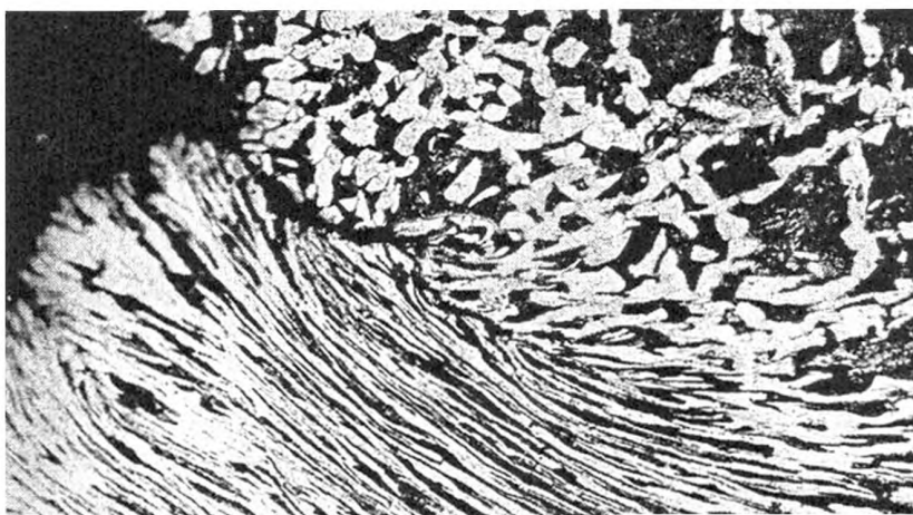
Рисунок А.1 — Микроструктура металла у намина (ув. 200 \times )
