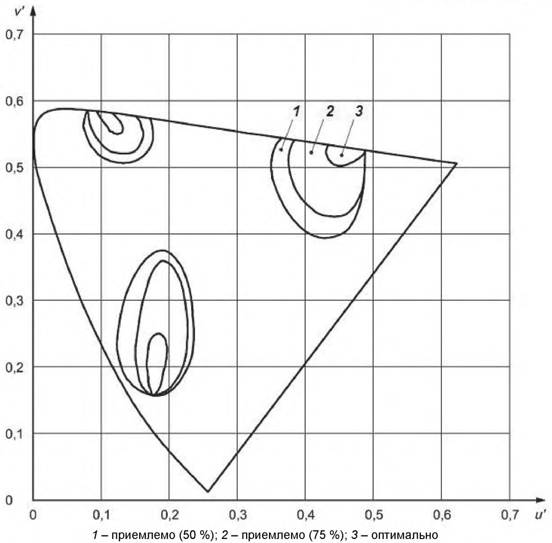
Рисунок 13 – Оптимальный и приемлемый цветовые диапазоны. Излучающие плоскпанельные ЖК-дисплеи
