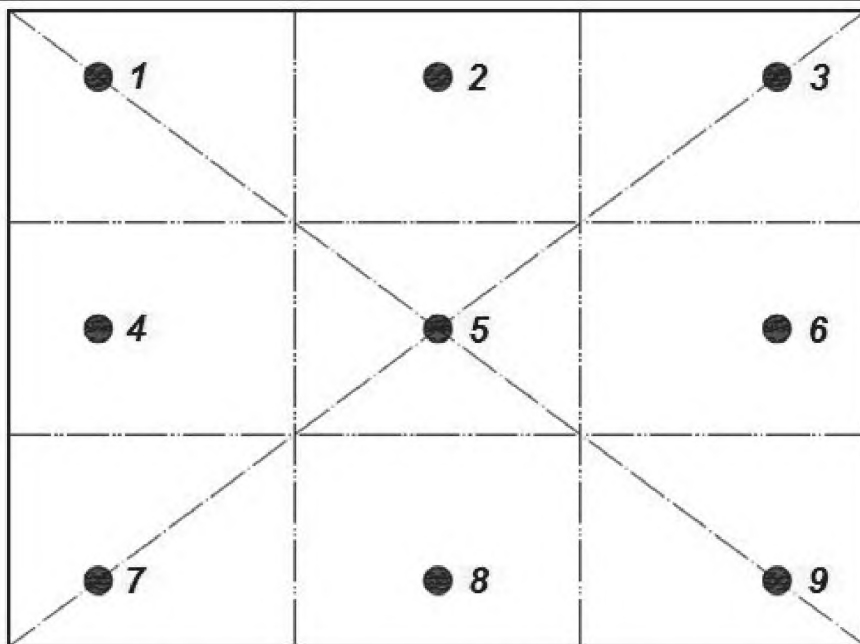
Рисунок 12 – Расположение точек измерений на анизотропном излучающем плоскостанельном ЖК-дисплее (преобладает реальная информация)
