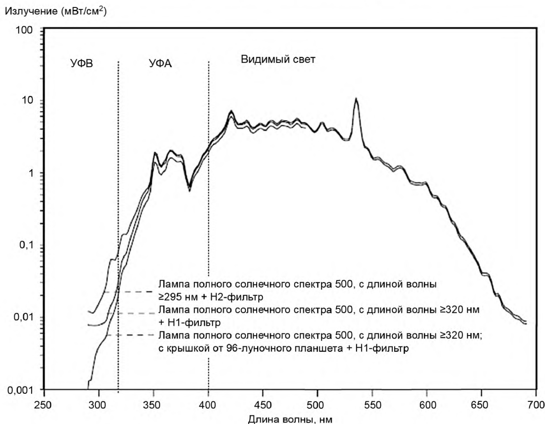
Рисунок 1 — Спектральное распределение излучения солнечного имитатора
