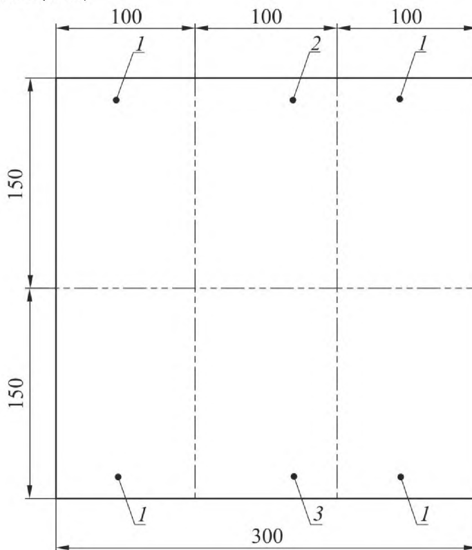
1 – образцы для испытаний; 2 – образец для визуального осмотра; 3 – образец для спектрофотометрического измерения
