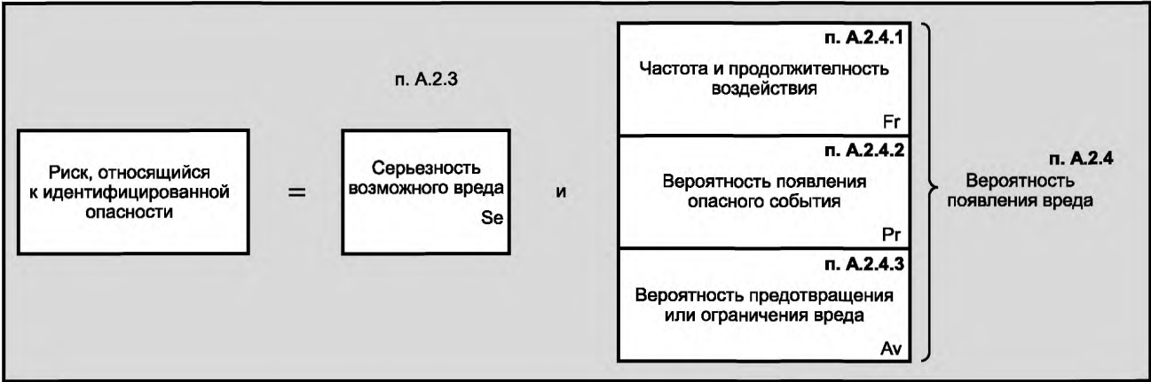
Рисунок А.2 — Параметры, используемые для оценки риска
