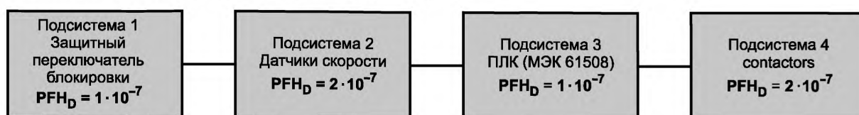
Рисунок В.8 — Оценка PFH_D для СБЭСУ
