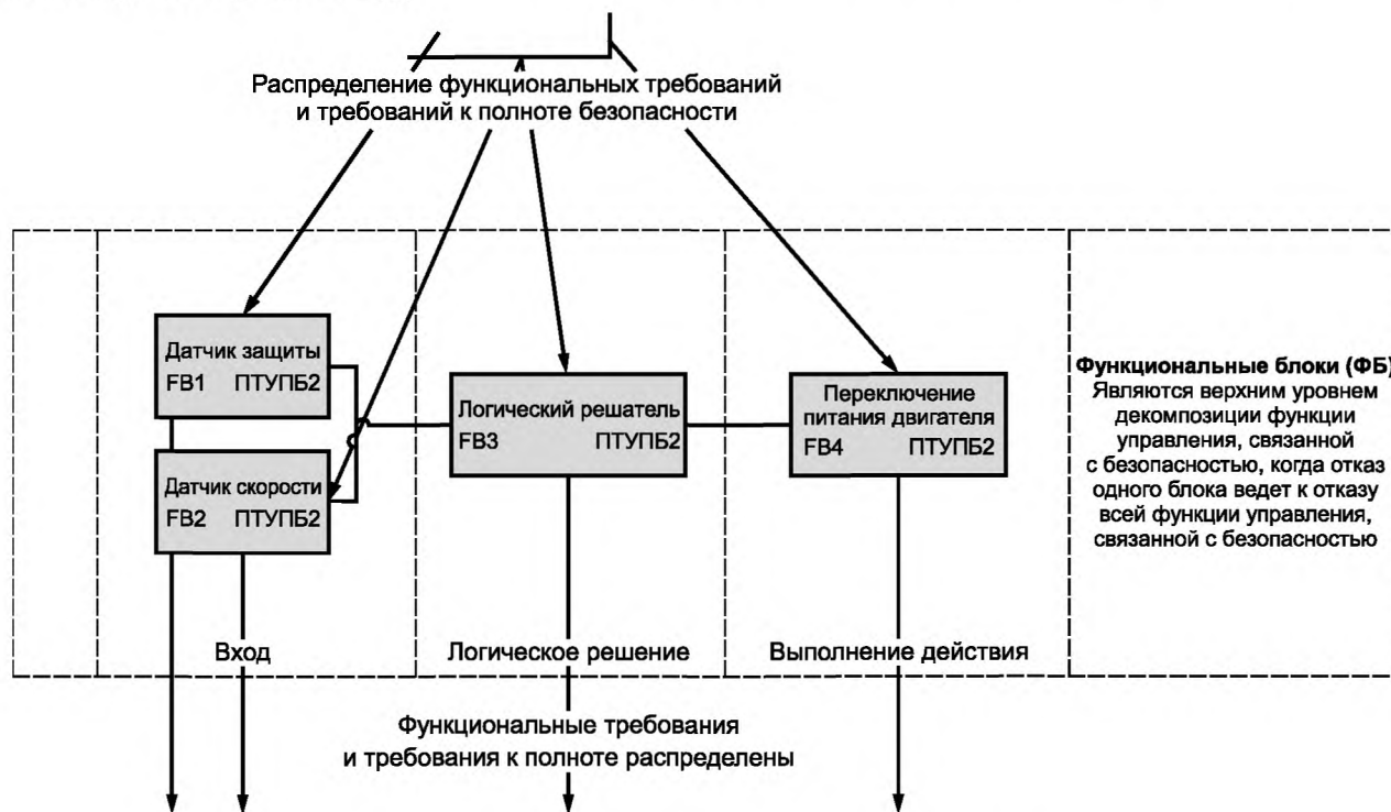
Рисунок В.5 — Начальная концепция архитектуры СБЭСУ
