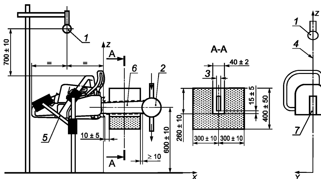
Рисунок А.1 — Испытательная установка для цепных пил
