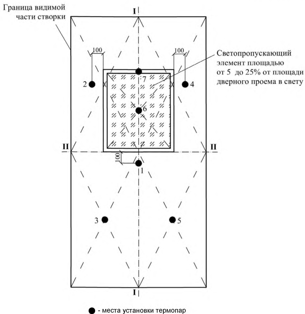
Рисунок А.2 - Схема установки термопар на необогреваемой поверхности створки одностворчатой распашной и горизонтально-раздвижной двери бокового открывания со светопрускающим элементом створки свыше 5 до 25% от площади дверного проема в свету
