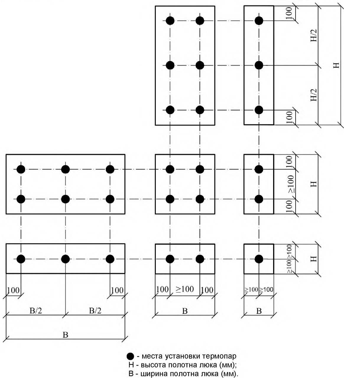
Рисунок А.5 – Схемы установки термодатчиков на необогреваемой поверхности люков площадью полотна, не превышающей 0,25 м 2
