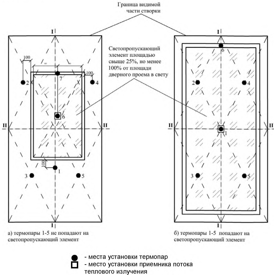
Рисунок А.3 - Схема установки термомпар и приемника потока теплового излучения на необогреваемой поверхности створки одностворчатой распашной и горизонтально-раздвижной двери бокового открывания со светопроницающим элементом створки свыше 25% но менее 100% от площади проема в свету
