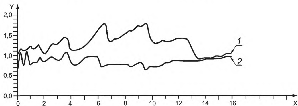
Рисунок D.3 — Нормированные значения площади поперечного сечения пучка при ограничениях FDA и МЭК для 5 преобразователей с различными ka при z = 0,5 см
