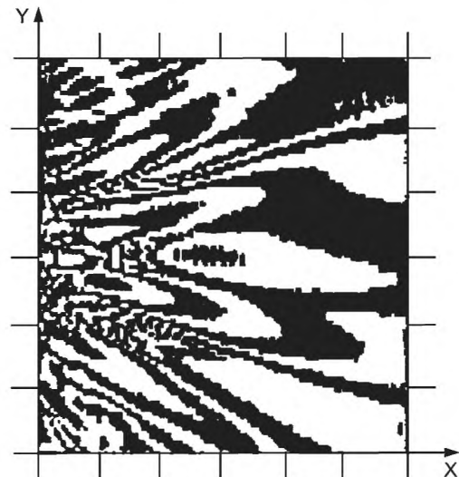
Рисунок D.1 — Линии равных давлений типовой физиотерапевтической лечебной головки малой геометрической площади ( a = 17 )
