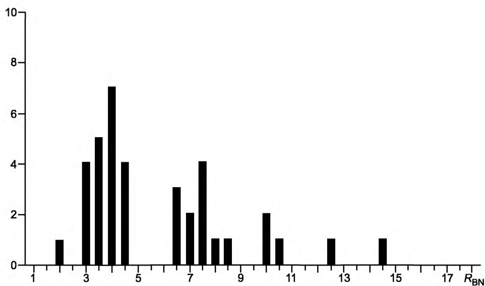
Рисунок А.2 Гистограмма распределений значений R_{\text{BN}} для 37 лечебных головок различных диаметров и частоты
