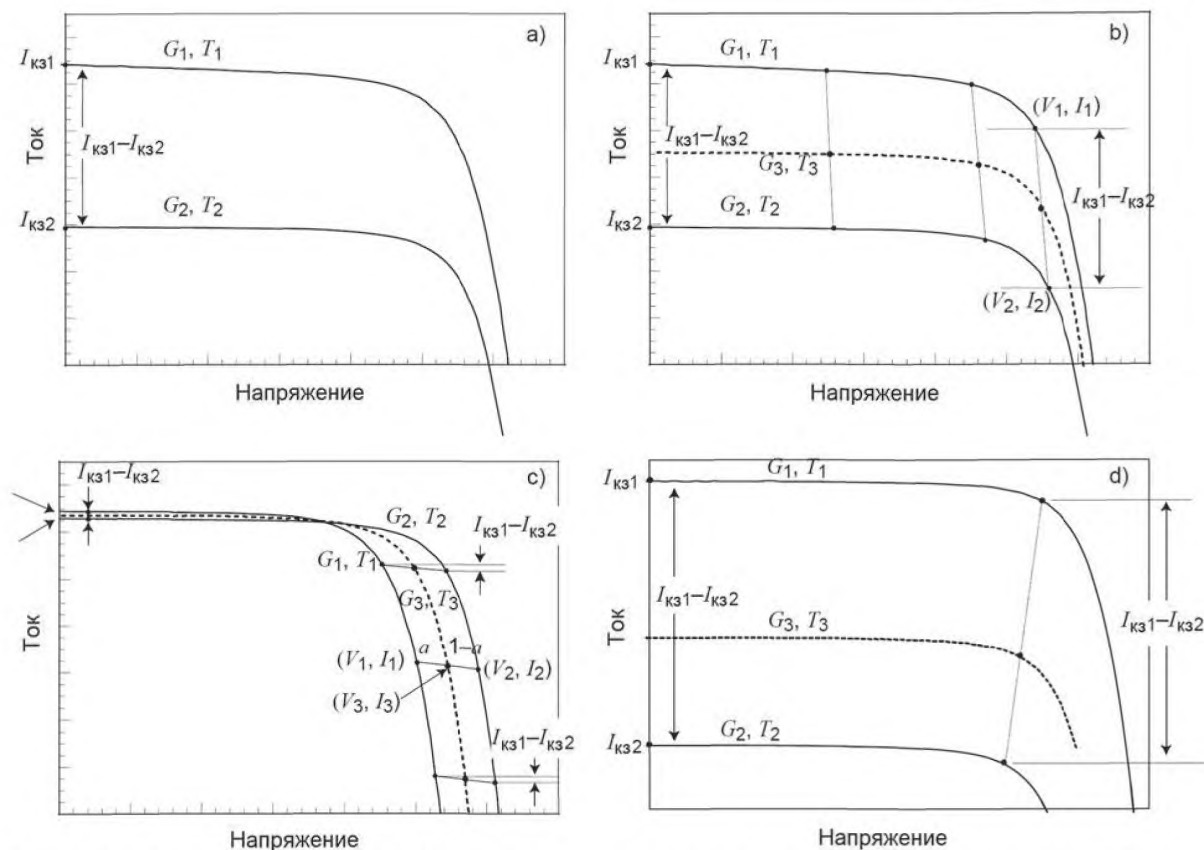
Рисунок 1 – Пример коррекции ВАХ с применением уравнений (6) и (7.) Рисунок (а) и (b) изображают коррекцию по энергетической освещенности, Рисунок (с) изображает коррекцию по температуре и Рисунок (d) – коррекцию одновременно по энергетической освещенности и температуре.
