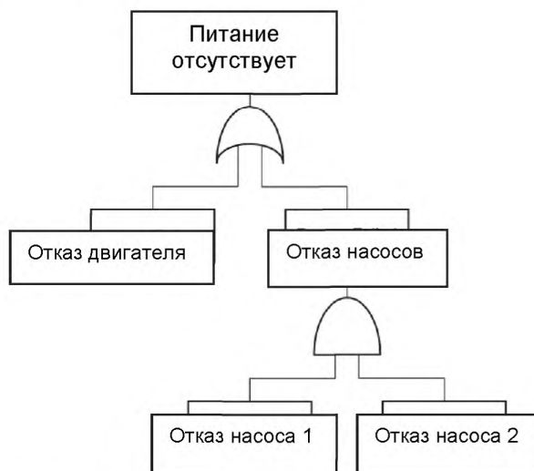
Рисунок В.1 – Дерево отказов для иллюстрации отказа в системе питания
