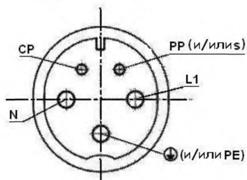
Расположение штырей (вид со стороны штырей)
