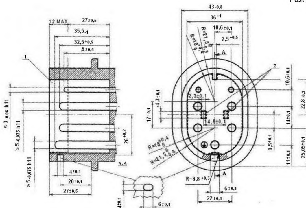
Конец штырей
