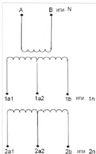
Рисунок 308 – Однофазный трансформатор с двумя многоотводными вторичными обмотками
