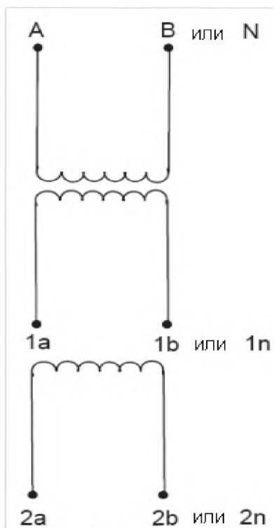
Рисунок 304 – Однофазный трансформатор с двумя вторичными обмотками
