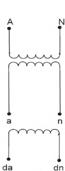
Рисунок 309 – Однофазный трансформатор с трансформатор с одной обмоткой напряжения нулевой последовательности
