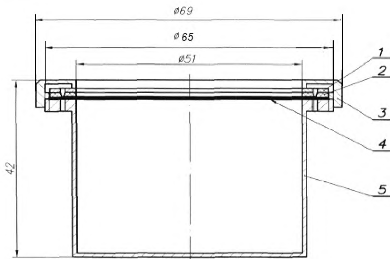
1 – металлическая уплотняющая прокладка; 2 – резиновая уплотняющая прокладка; 3 – крышка; 4 – образец материала; 5 – металлический стакан
