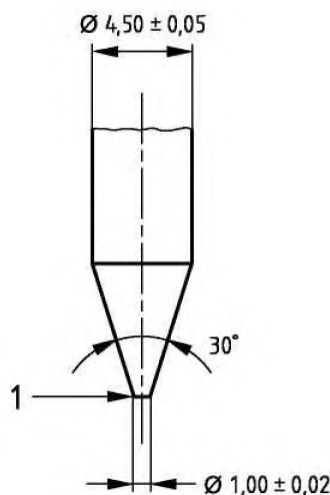
Рисунок 10 — Испытательный гвоздь для определения сопротивления проколу
