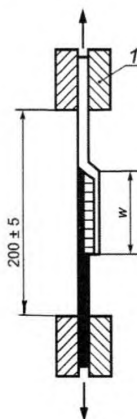
1 – зажим; w – ширина клеевого соединения
