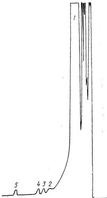
1 – этилбензол; 2 – диэтилбензол; 3 – m -этилизопропилбензол; 4 – додекан; 5 – гексадекан; (3,4,5 – внутренний эталон, используют любой из указанных углеводородов)
