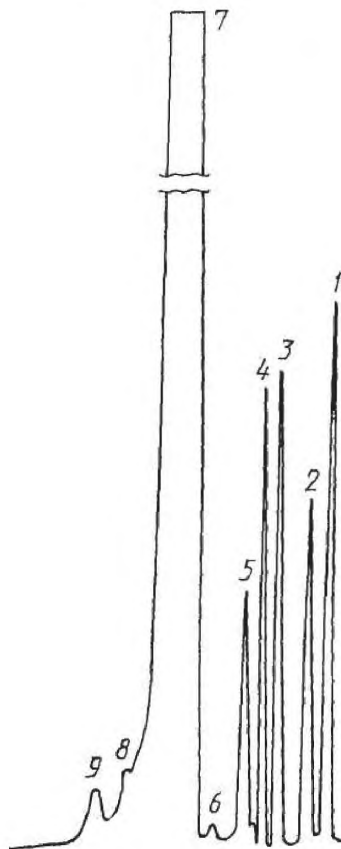
1 – n -гексан (внутренний эталон); 2 – бензол; 3, 5, 6 – парафиновые углеводороды; 4 – толуол; 7 – этилбензол; 8 – o -ксилол; 9 – изопропилбензол
