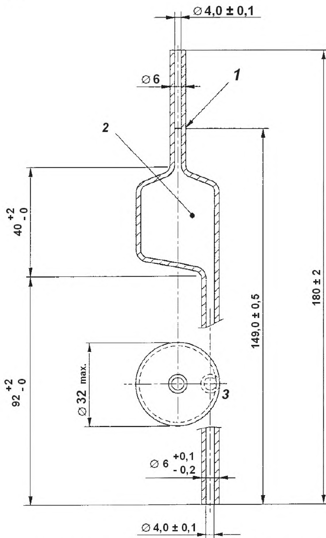
1 – метка; 2 – вместимость пипетки до метки – (20,0 \pm 0,2) \text{ см}^3 ; 3 – сечение Рисунок 6 – Пипетка
