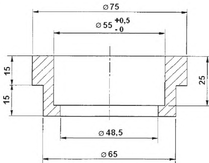
Рисунок 4 – Поддерживающее кольцо
