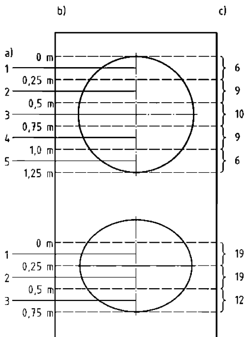
Рисунок 7 – Типовые схемы отбора проб для полного цилиндрического резервуара и частично заполненного бака овальной сечения
