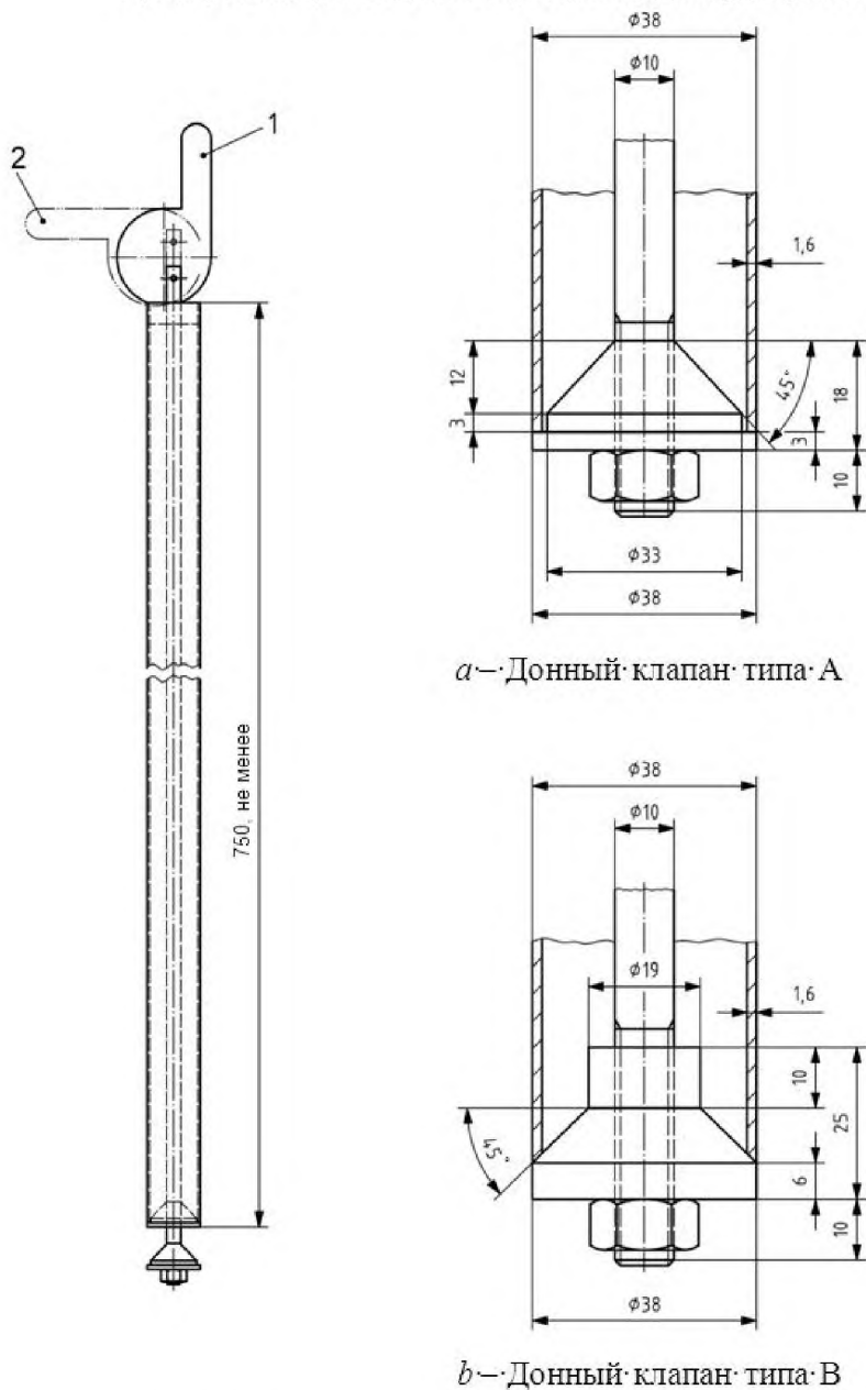
Рисунок D.1 — Стандартная пробоотборная трубка
