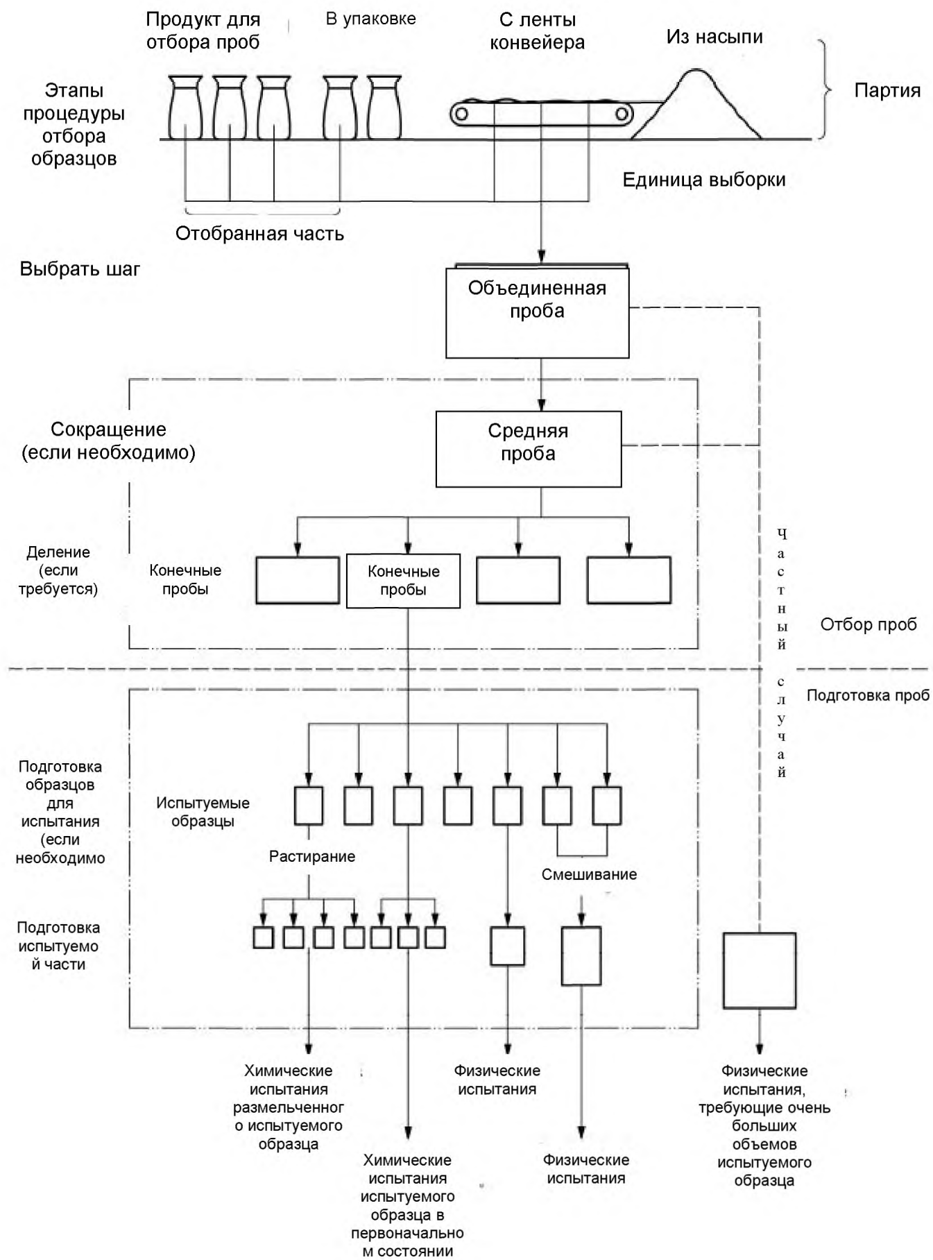
Рисунок 1 —Схема отбора проб твердых веществ
