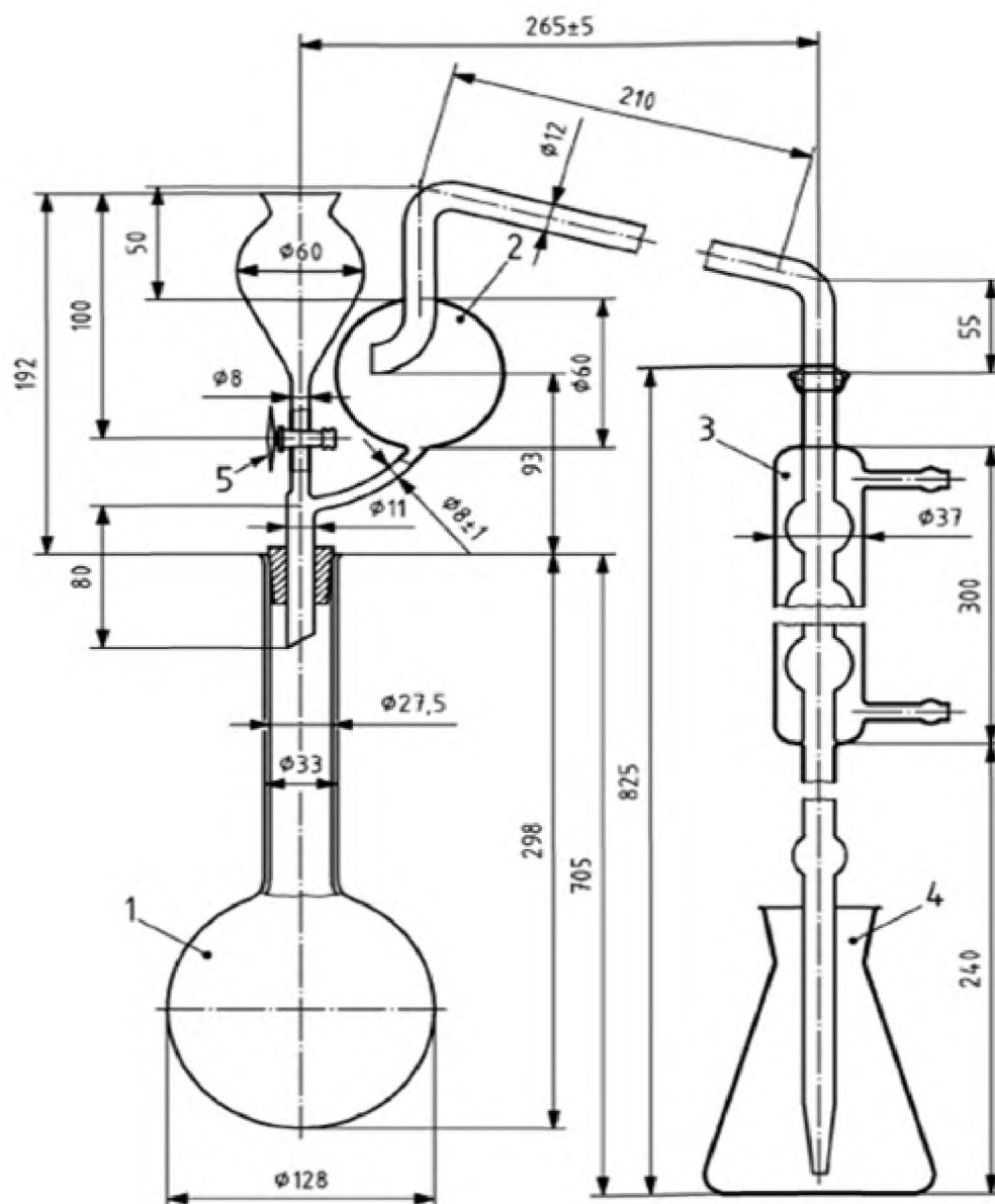
Рисунок 3 — Перегонный аппарат 3
