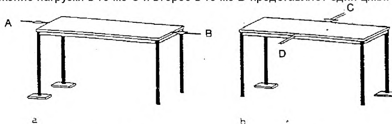
Рисунок 2 – Приложение нагрузки и расположение упоров при испытании горизонтальной статической нагрузкой
