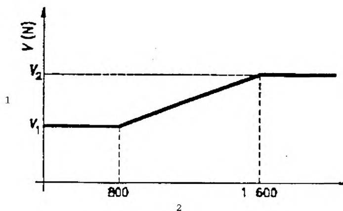
1 – вертикальная нагрузка; 2 – максимальный размер крышки стола в направлении возможного опрокидывания. Рисунок 6 – Определение вертикальной статической нагрузки
