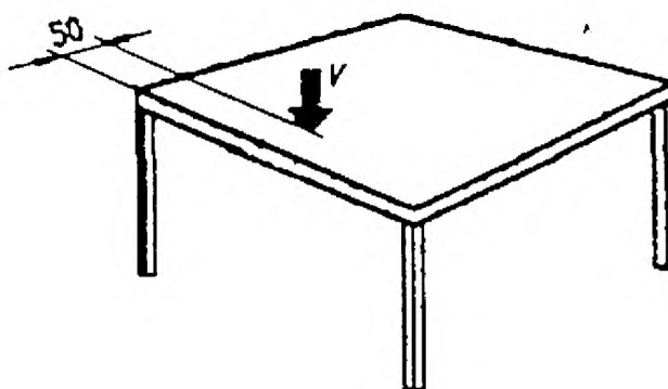
Рисунок 7 – Испытание на устойчивость под действием вертикальной нагрузки
