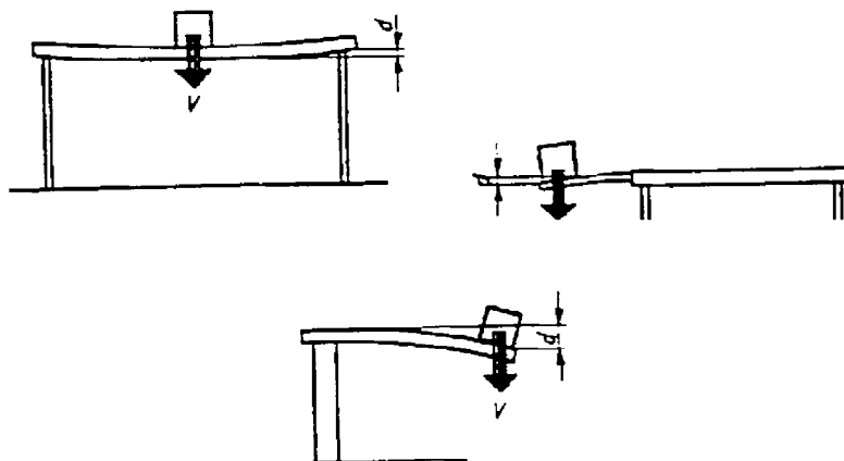
Рисунок 4 – Испытание на прочность под действием вертикальной статической нагрузки
