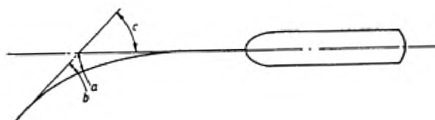
Рисунок Г.2 - Определение угла остаточной деформации
