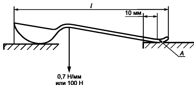
Рисунок 1 — Испытание ложки на прочность
