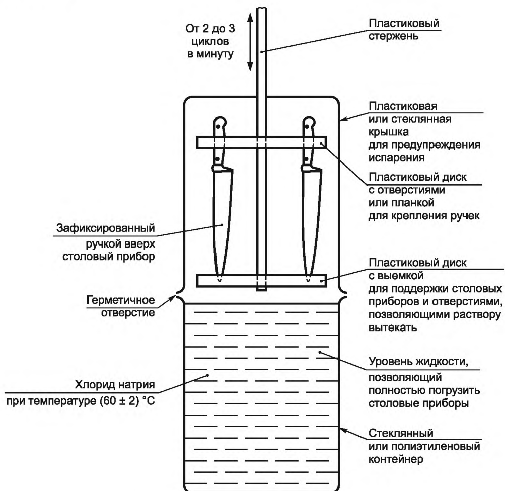
Рисунок С.1 — Оборудование для коррозионных испытаний
