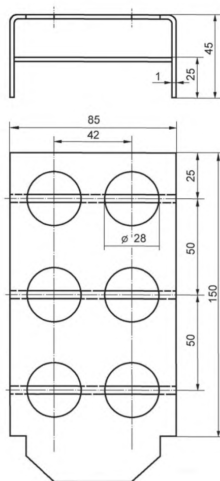
Рисунок 4 — Подставка для шести тиглей
