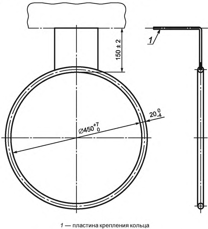
Рисунок 11 — Размеры баскетбольного кольца
