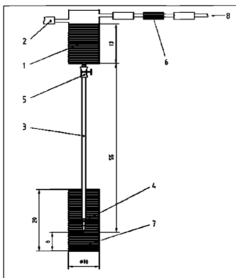
Рисунок 1 – Установка для отмывания примесей
