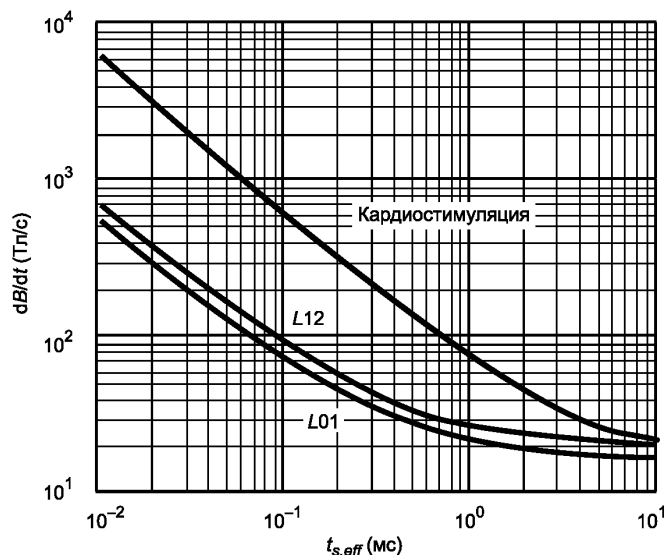
Рисунок 201.102 — ПДУ для случаев кардиостимуляции и ВПНС
