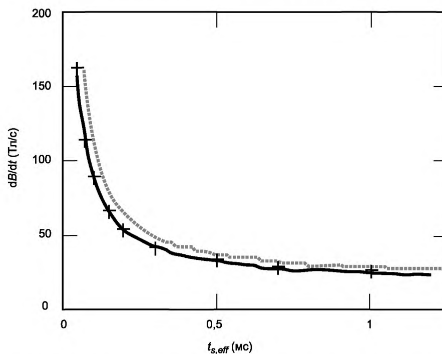
Рисунок АА.5 — Профиль градиента G , сигнал стимула dB/dt и значение ответной реакции R для трапецеидального EPI профиля с началом в точке t = 0
