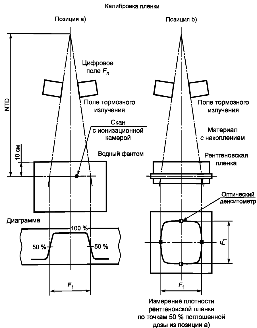
Рисунок 9 — Испытания по 10.1.1.3
