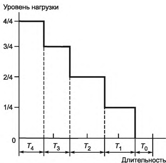
Рисунок С.3 — Пример графика длительности нагрузки
