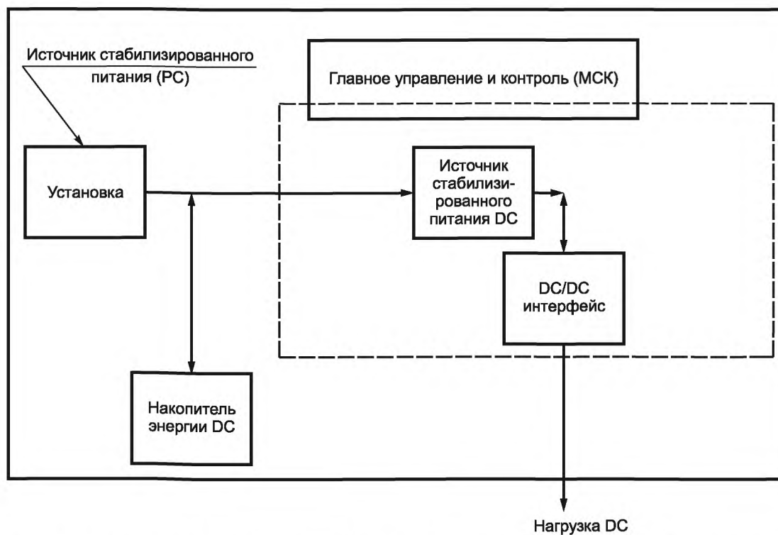
Рисунок А.3 — Конфигурация источника стабилизированного питания с постоянным током на выходе, принятая для измерения КПД
