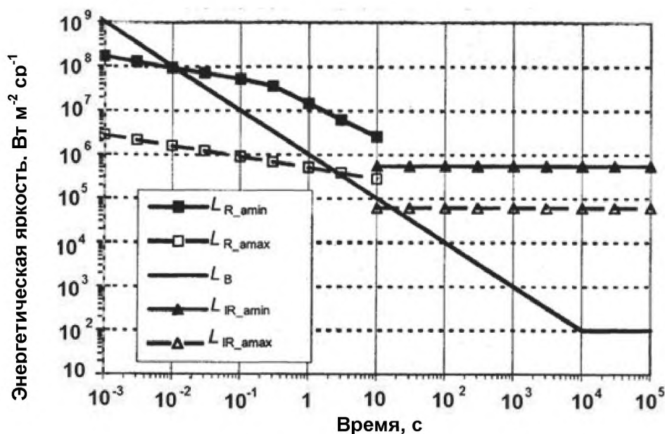
Рисунок 5.5 – Зависимость пределов облучения взвешенной энергетической яркости от времени для постоянного облучения
