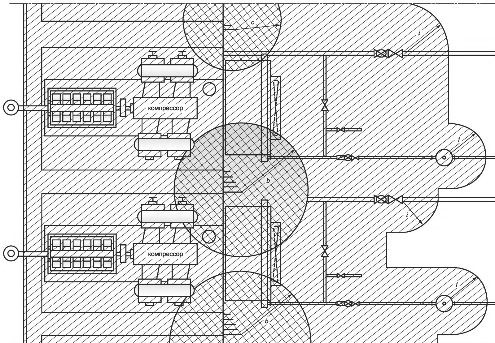
Рисунок D. 1a — Пример классификации зон для компрессора, работающего на природном газе
