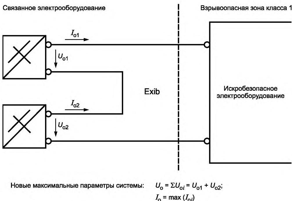
Рисунок I.1 — Последовательное соединение.
