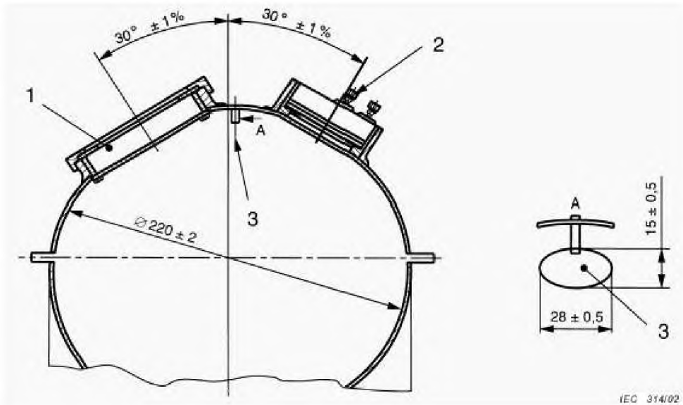
1 - апертура фары 2 - фотоэлемент 3 - дефлектор А – увеличение (расширение) дефлектора (вид в направлении стрелки)
