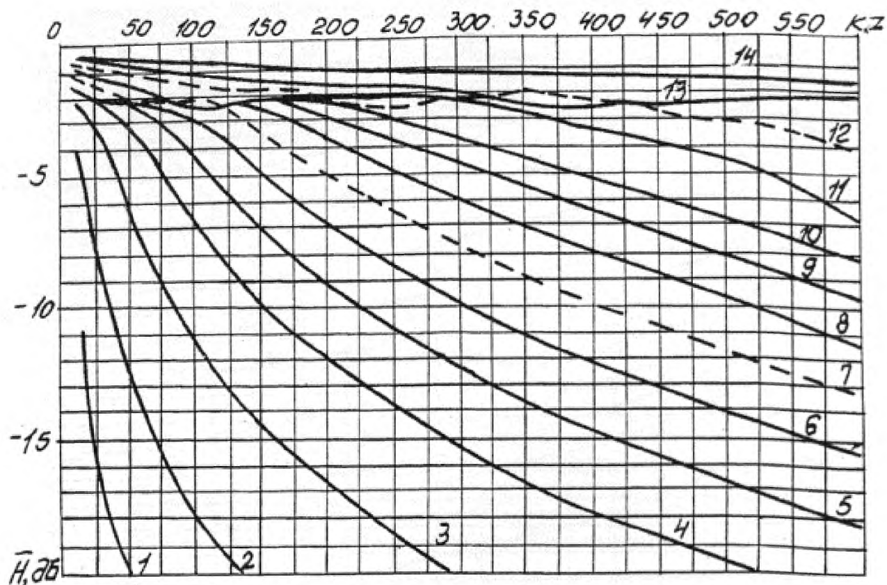
Рисунок 20 — Значения параметра взаимности \bar{H} для ПЭП с круглой пьезопластиной, нагруженного на сталь 45
