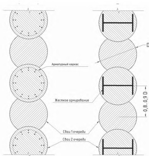
Рисунок 1 – Буресекующие сваи, схема армирования
