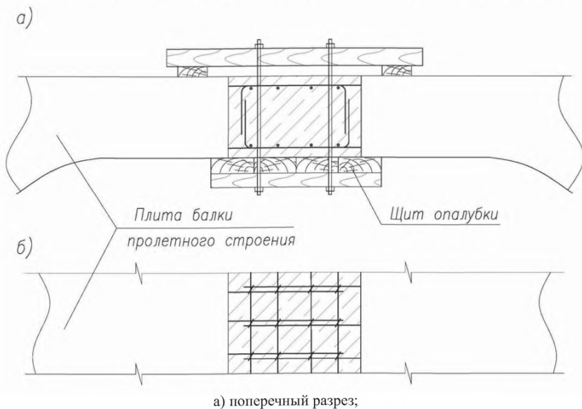
Рисунок 4 – Схема стыка блоков пролетных строений
