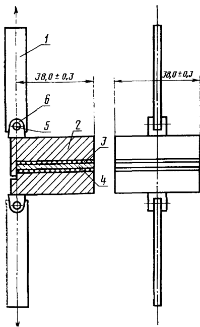
1—хвостовик; 2—колотка; 3—склеивающая лента; 4—образец картона; 5—серьга
