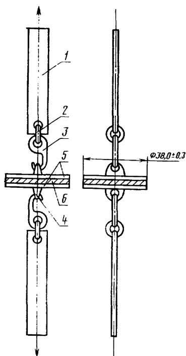
1—хвостовик; 2—кольцо; 3—серьга; 4—ушко; 5—стальные пластинки; 6—об- разец картона
