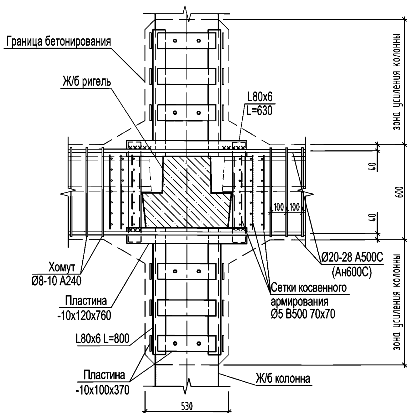
Рисунок 6.18 – Устройство монолитного продольного ригеля
