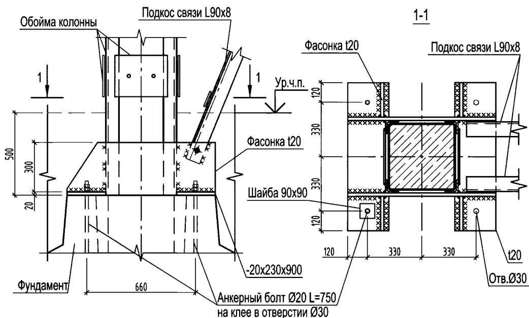
Рисунок 6.4 – Крепление подкоса стальных связей к фундаменту
