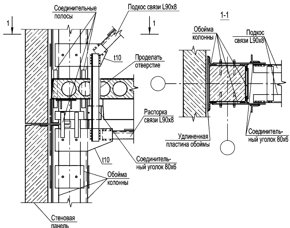
Рисунок 6.3 – Крепление поперечных связей к стальной обойме колонны
