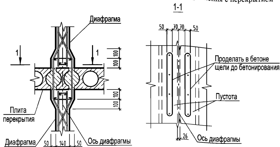
Рисунок 6.8 – Соединение диафрагм продольного направления с перекрытием из многпустотных плит
