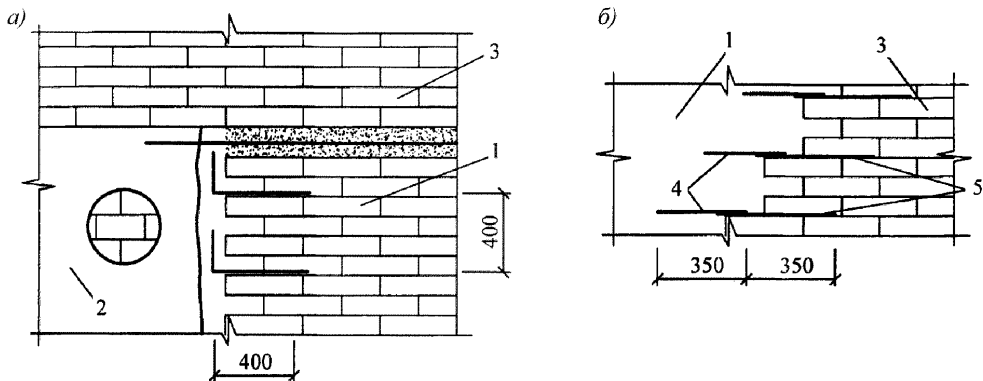
а ) – при поэтапной кладке; б ) – при соединении со старой кладкой
