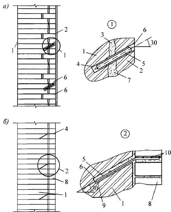
а) – с установкой стальных связей; б) – заменой облицовки путем крепления анкерами с существующей кладкой
