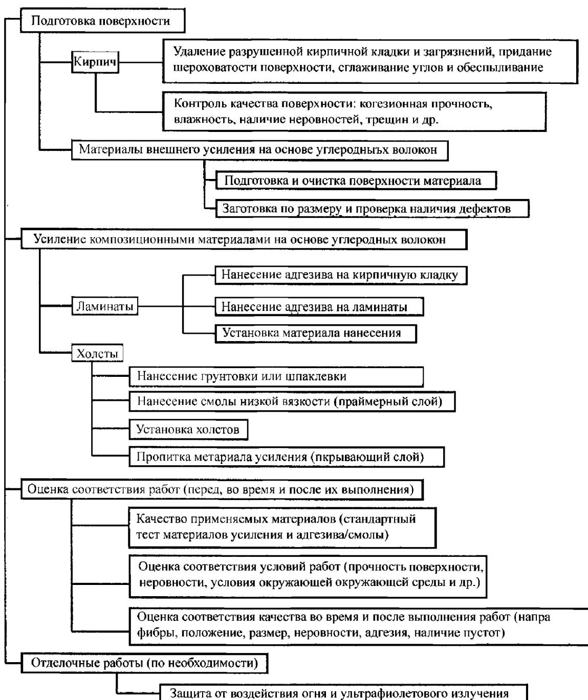
Рисунок 35 – Технологическая схема внешнего армирования кирпичных конструкций композиционными материалами
