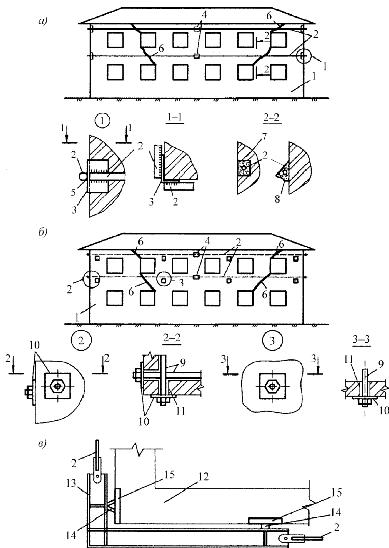
а) – с наружной стороны стен; б) – то же с внутренней стороны; в) – с центрирующими элементами по углам
