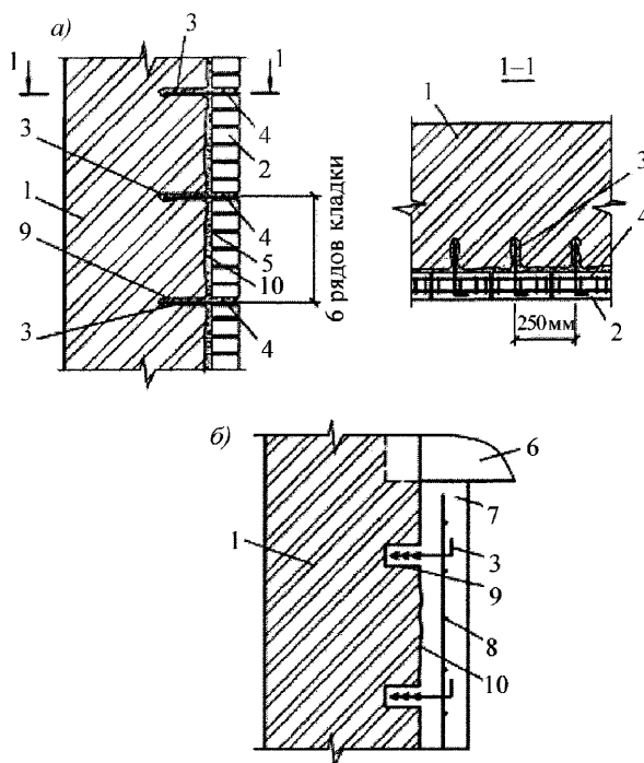
а) – прикладкой; б) – набетонкой
