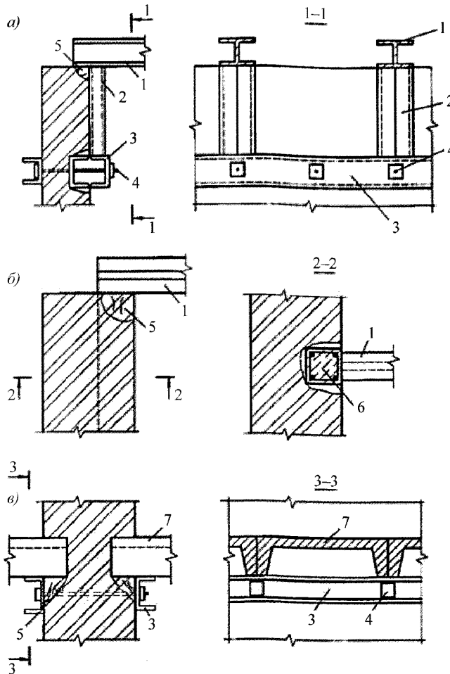
а) – короткими стойками; б) – врезной стойкой; в) – стальным поясом
