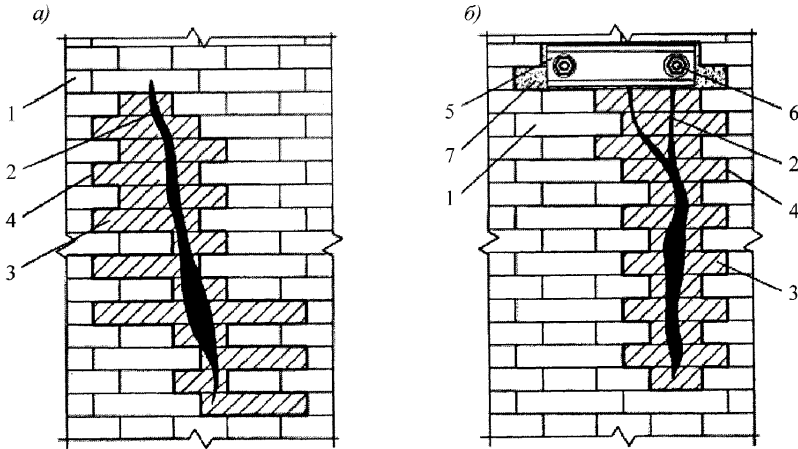
а ) – с широкими трещинами вставкой простых кирпичных замков; б ) – то же вставкой кирпичных замков с якорем
