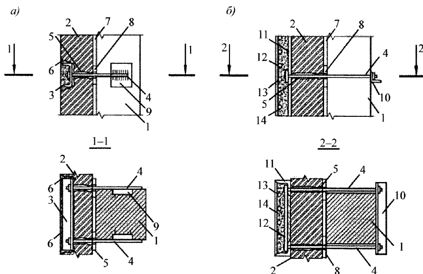
а) – через швеллер углубленный в стену; б) – через накладные уголки
